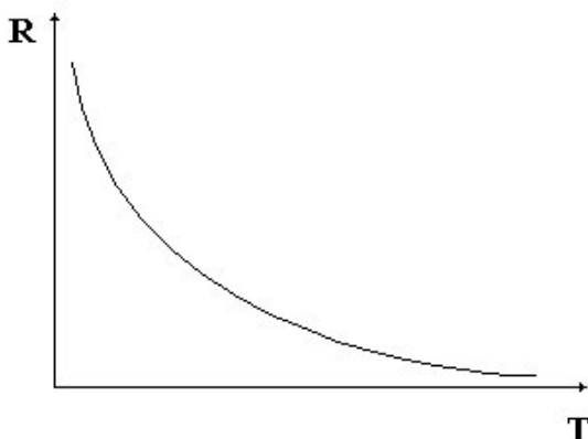
Fig. 2 Caracteristica termică a termistorului NTC.
